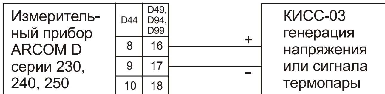
Рис.7.4. Схема подключения входных каналов для измерения сигналов ТП
