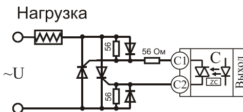
Подключение внешних тиристоров к выходу "С"
