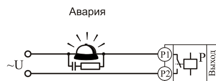
Подключение аварийной сигнализации к выходу "Р"
