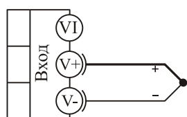
термопара
