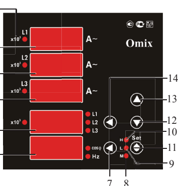
Рис. 1 – Управляющие элементы
