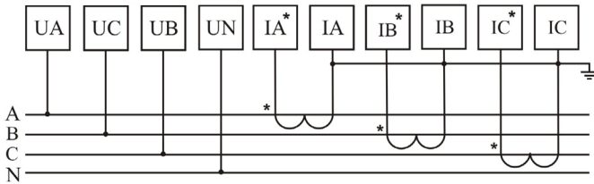
Рис. 7 – Подключение трансформатора тока (трехфазная цепь с нейтралью)
