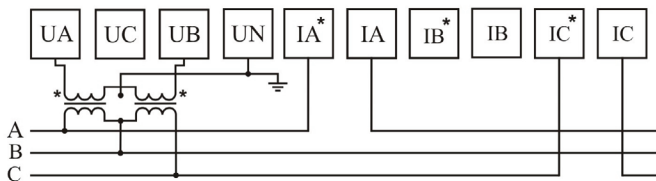
Рис. 10 – Подключение трансформатора напряжения (трехфазная цепь без нейтрали)
