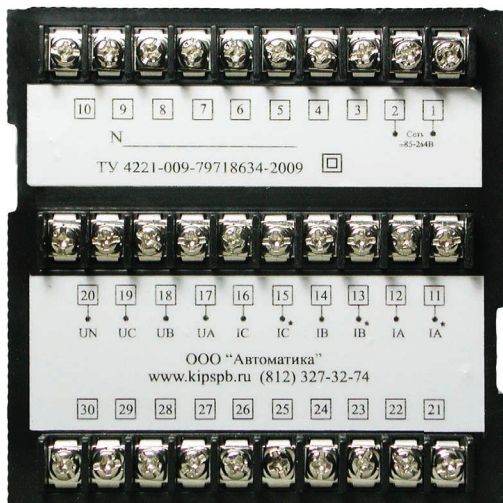
Рис. 13 – Задняя панель прибора
