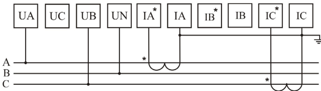
Рис. 8 – Подключение трансформатора тока (трехфазная цепь без нейтрали)
