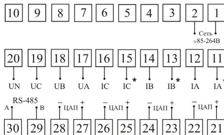
Рис. 4 – Клеммы подключения
