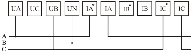
Рис. 6 – Подключение напрямую (трехфазная цепь без нейтрали)
