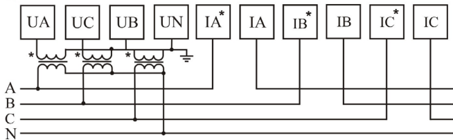
Рис. 9 – Подключение трансформатора напряжения (трехфазная цепь с нейтралью)
