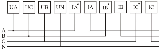
Рис. 5 – Подключение напрямую (трехфазная цепь с нейтралью)
