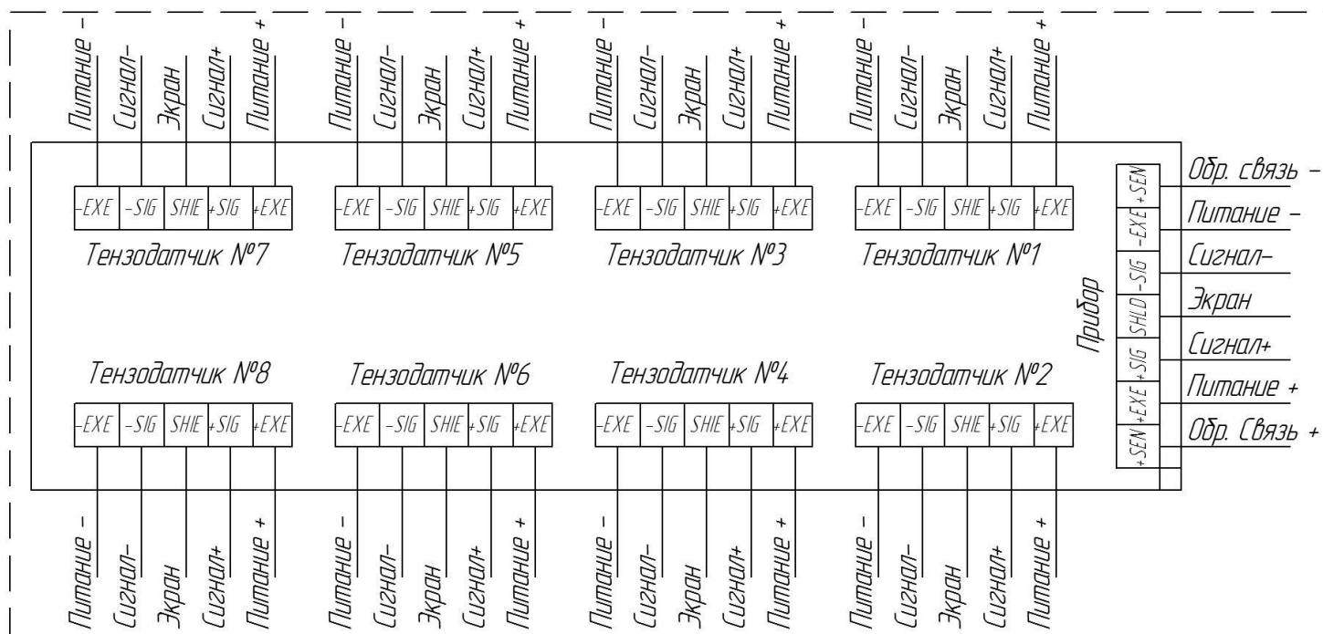
Маркировка клемм подключения тензодатчиков
