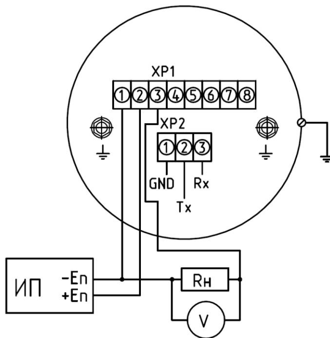
Рисунок В.10 – Прибор ДМ5002Вн-Б
