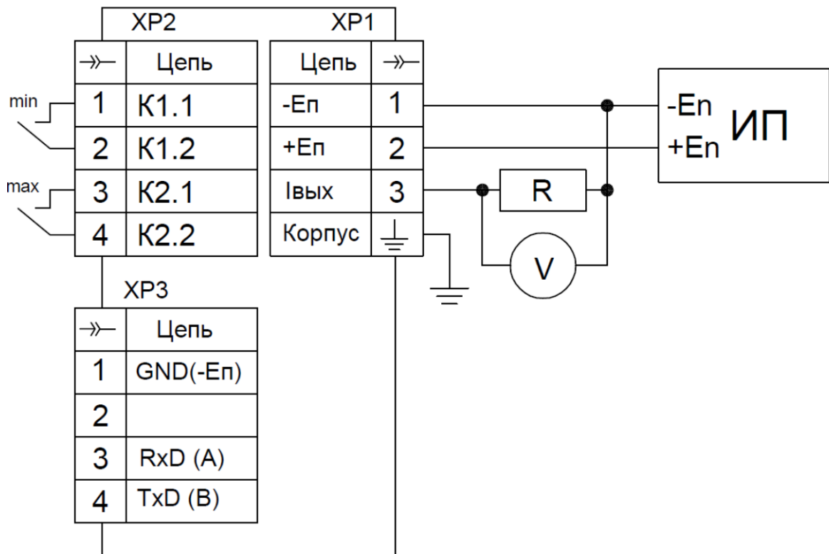
Рисунок В.7 – Прибор ДМ5002М-Г
