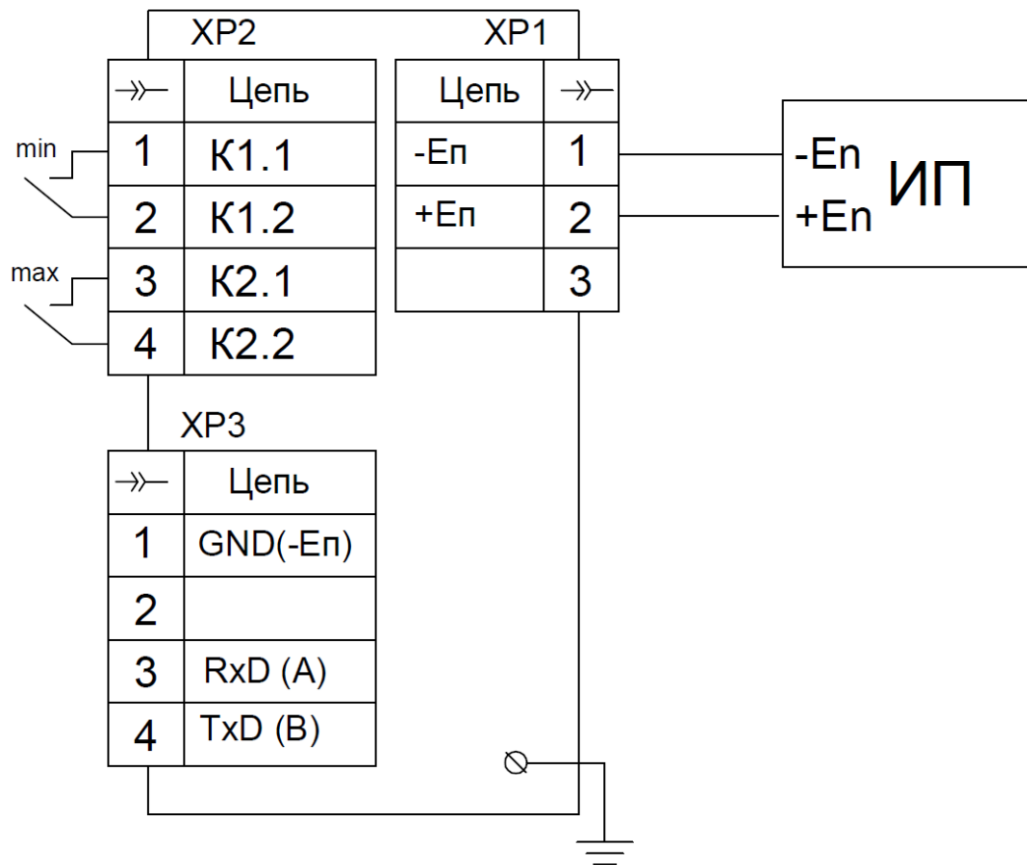
Рисунок В.6 – Прибор ДМ5002М-В-А
