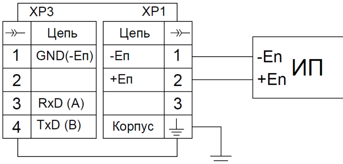
Рисунок В.1 – Прибор ДМ5002М-А
