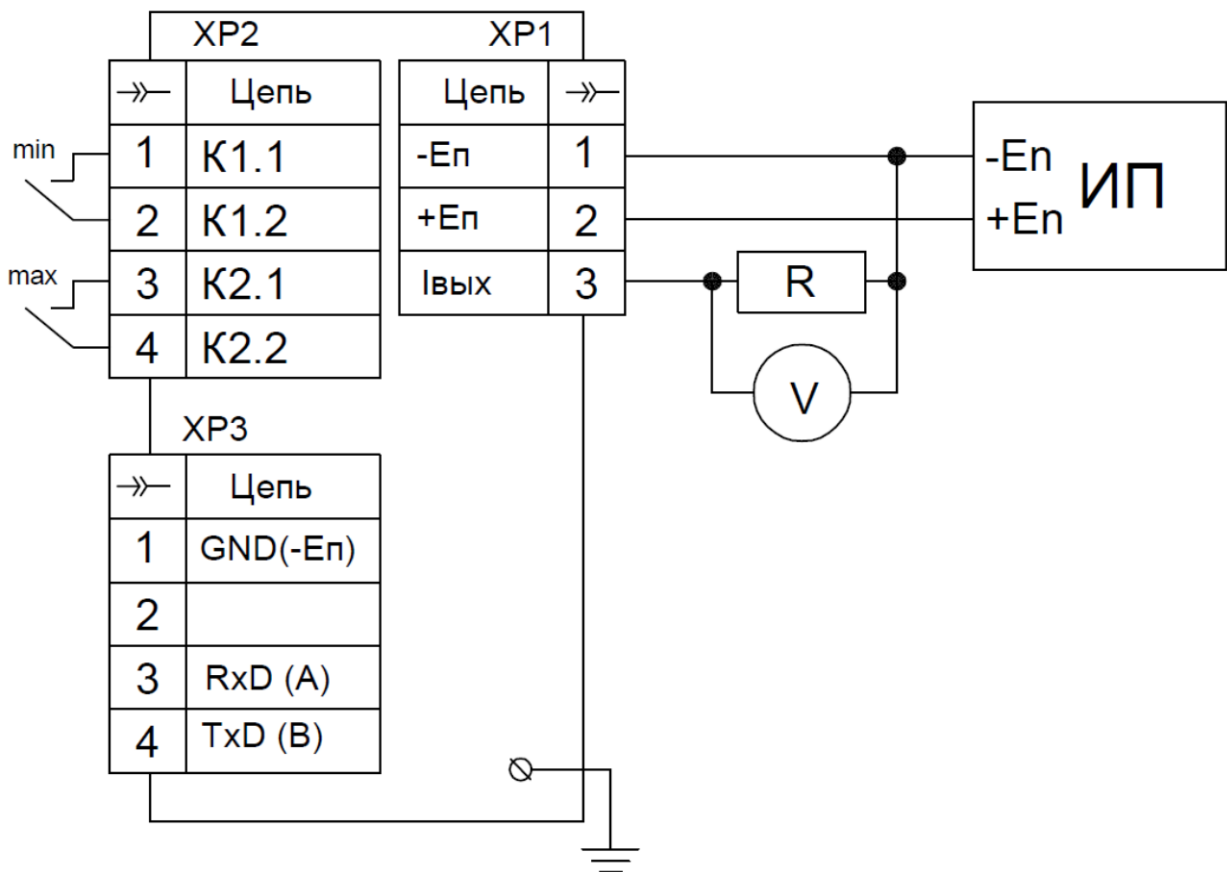
Рисунок В.8 – Прибор ДМ5002М-Г-А
