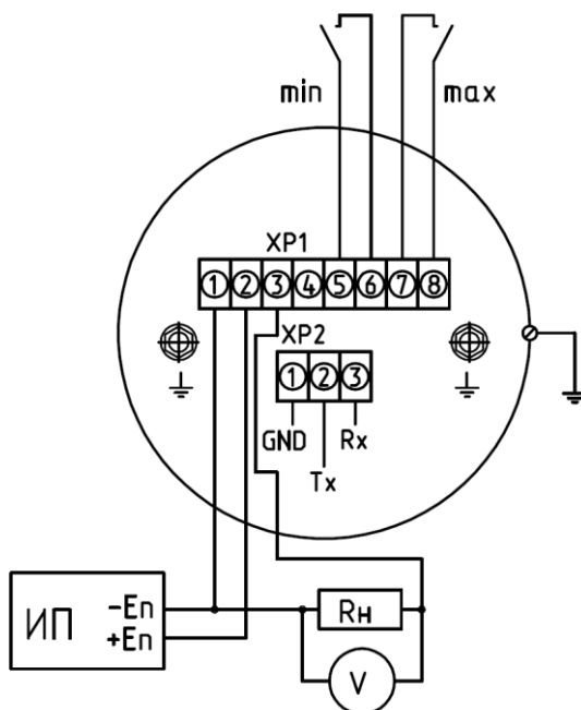
Рисунок В.12 – ДМ5002ВН-Г
