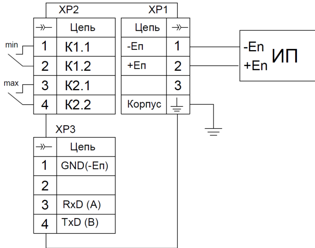
Рисунок В.5 – Прибор ДМ5002М-В
