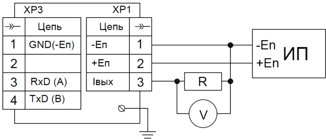
Рисунок В.4 – Прибор ДМ5002М-Б-А
