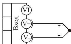
термопара
