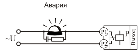
Подключение аварийной сигнализации к выходу "P"
