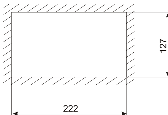
Вырез в щите
